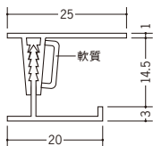
40020 湯らっくす 不燃用廻り縁 3m / アルミ製 (ベース: ビニール) 焼付塗装
