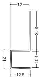
20071 ステン SZ-12 2.73m/ヘアライン t=0.8mm
