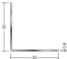
20033 ステンアングル 0.8×30×30 3m/ヘアーライン
