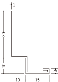
31086 PFL-150 2m/ホワイト/50本入
