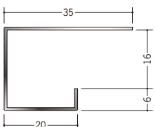
20166 ステン STC-1620 3m/ヘアライン/t=0.8mm
