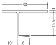
34326 CAP-1510 1.82m/ホワイト/100本入
