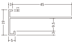
33527 FCX-9.5M (岩綿板用) 2m/ホワイト/50本入
