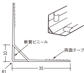
01301 クッションコーナー1型 テープ付 2.5m/ミルキー/50本入
