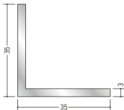
56130 アルミアングル 3×35×35 3m / アルマイトシルバー
