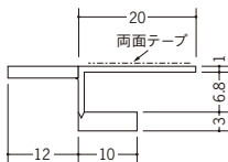
33017 FS-6 テープ付 1.82m/ホワイト/30本入
