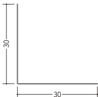
63185 L-30 1.82m / アエンメッキ鋼板 t=0.27mm
