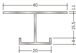
59093 アルミ天井織手15型 アクリル焼付 3m / ネオシルバー・ネオステンカラー
