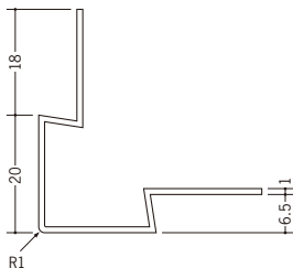
37125 角型イカ出隅6.5 2.73m/ホワイト/50本入
