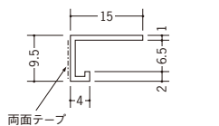
31006 PSD-6 テープ付 2.3m/ホワイト/140本入
