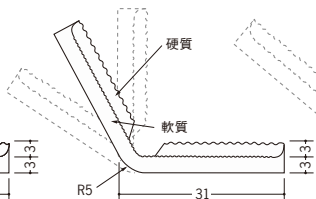
09022 ソフトコーナー31 2.73m/ミルクイー/12本入
