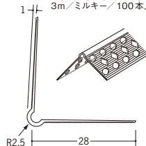
04080 コーナービート28穴あき 2.5m/ミルキー/100本入 3m/ミルキー/100本入
