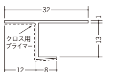
34032 CP-12 1.82m/ホワイト/100本入
