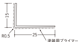
01314 L型コーナー15×25 プライマー付 2.5m/ミルキー/100本入 2.73m/ミルキー/100本入
