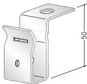
65020 ワンタッチハンガー (H=50) t=2.0mm / 300コ入
