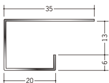
20165 ステン STC-1320 3m/ヘアライン/t=0.8mm
