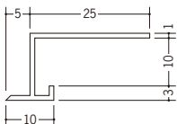
33076 SLP-9.5 1.82m/ホワイト/100本入
