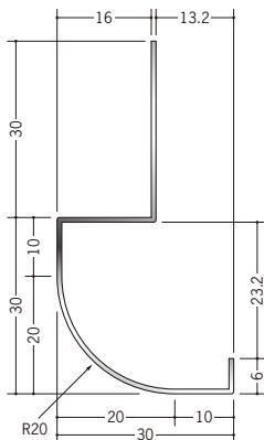
20098 ステン LER-1520 2.73m/ヘアーライン t=0.8mm
