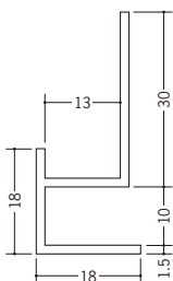
31078 CMX-0912 2m/ホワイト/50本入
