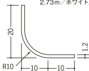
01190 ビニール 10R-20×20 1.82m/ホワイト/100本入 2.73m/ホワイト/100本入
