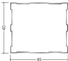
65048 角スタット4045 3m/ t=0.5mm/ 10本束
