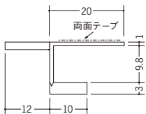
33018 FS-9 テープ付 1.82m/ホワイト/25本入
