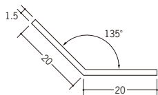
36152 角度付アングル20 2.73m/ホワイト/100本入
