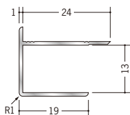
50078 アルミ 12AD 2.73m/アルマイトシルバー 3m/アルマイトシルバー
