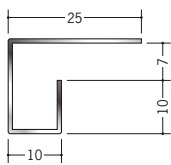
20172 ステン STC-710 3m/ヘア-ライン/t=0.8mm
