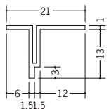
34066 GT-13 1.82m/ホワイト 150本入
