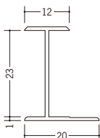
35103 HG-23 1.82m/ホワイト/50本入 2.42m/ホワイト/50本入
