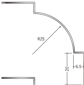
64101 ステン IR-625 2.73m/ヘアライン・鏡面 (#800) t=0.8mm
