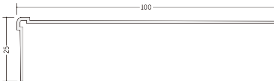
08020 養生アングル25×100 1.5m / イエロー / 塩化ビニール 50本入
