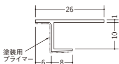
33304 PPZ-906 2m/ホワイト/100本入
