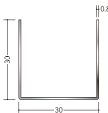
20024 ステンチャンネル 0.8×30×30 3m/ヘアーライン
