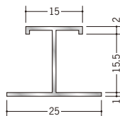
54115 アルミ EH-16 3m/アルマイトシルバー
