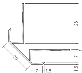
53011 アルミ DAM-1320 2.73m / アルマイトシルバー
