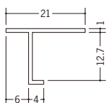
33105 TV-612 1.82m/ホワイト/150本入
