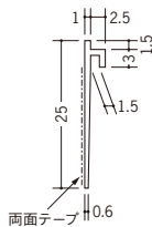
33311 クロス押さえ見切1型-A テープ付 2m/ホワイト/150本入
