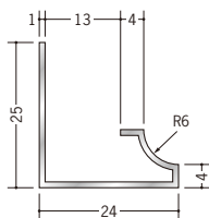
52004 アルミRSA-12 3m / アルマイトシルバー
