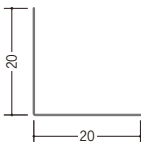
63183 L-20 1.82m / アエンメッキ鋼板 t=0.27mm
