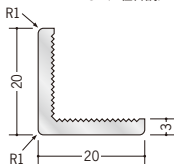
36312 木目アングル20出隅用 2.5m / 枠目調 / 50本入
