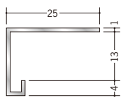
52026 アルミCC12 3m / アルマイトシルバー
