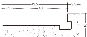
01345 袖壁コーナー 40-9 (9.5mm用) 2.6m/ミルキー/20本入
