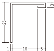
33176 HKT-15S 1.82m/ホワイト 100本入
