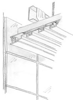
60081 廻り縁KS-15型 アクリル焼付 3m/焼付塗装 ベース (ビニール)/クリーム・グレー・ブラウン
