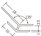
37109 出隅 135°-3 2.5m/ホワイト/50本入 2.73m/ホワイト/50本入
