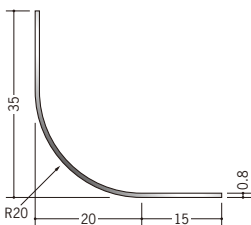
20067 ステンアングル SL35-20R 3m/ヘアーライン
