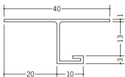
33250 換気見切 KMK-13 1.818m / ホワイト / 50本入 / 開口率11.96%
