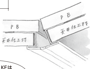
37015 フリージョイナージョイント
