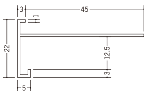
33528 FCX-12.5M (岩綿板用) 2m/ホワイト/50本入
