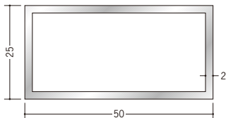
56331 アルミ角パイプ 2×25×50 2.5m (-3mm, +5mm) アルマイトシルバー
