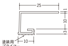
33207 ペンキ見切コ型10 2m/ホワイト/100本入
