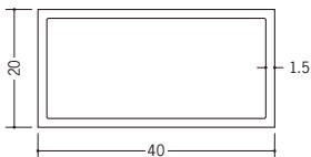
36074 角パイプ20×40 2m/ホワイト/40本入
