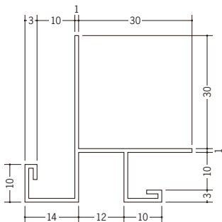
31110 DS-1212 2m/ホワイト/30本入
