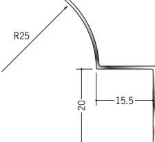
64104 ステン IR-1525 2.73m/ヘアライン・鏡面 (#800) t=0.8mm
