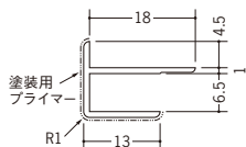
39077 ペンキ出隅 6.5 2.73m/ホワイト/100本入
