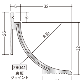
55047 アルミCR-2 (巾木) 3m/アルミトシルバー
