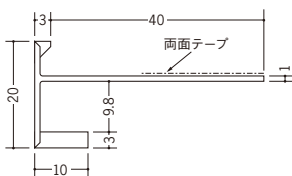
31013 EF-15 テープ付 2m/ホワイト/50本入
