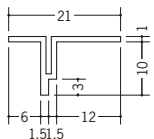
34065 GT-10 1.82m/ホワイト 150本入
