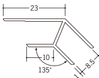
37043 入隅 135°-9 2.5m/ホワイト/50本入 2.73m/ホワイト/50本入
