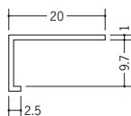
37523 TSC-9 2m/ホワイト/100本入
