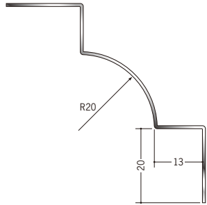
64073 ステン IR-1220 2.73m/ヘアライン・鏡面 (#800) t=0.8mm
