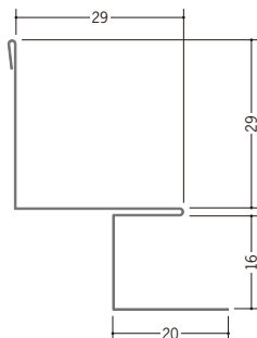
63161 亜鉛入隅 15B 1.82m / アエンメッキ鋼板 t=0.27mm
