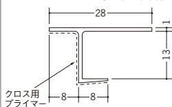
34355 CP-1208 1.82m/ホワイト/100本入
