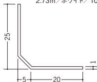
01131 ビニール面取 L25-5M 1.82m/ホワイト/100本入 2.73m/ホワイト/100本入
