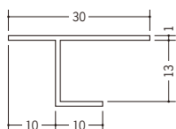
37534 TZT-12 2m/ホワイト/100本入
