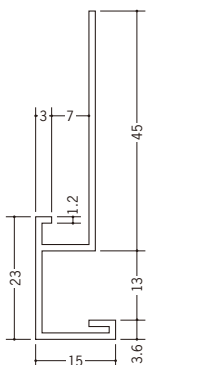
31058 CX-1206 2m/ホワイト/50本入
