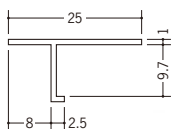
33288 TXV-9 2m/ホワイト/100本入
