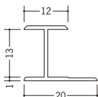
35037 HG-12.5 1.82m/ホワイト/50本入 2.42m/ホワイト/50本入
