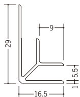
35024 カラー入隅5 2.73m/各50本入 下記全色あり
