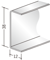
65003 C型チャンネル38 1.5m・3m / t=1.0~1.1mm 各10本束
