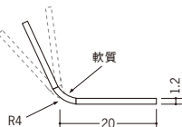
36144 フリーアングル30 2.5m/ホワイト/60本入
