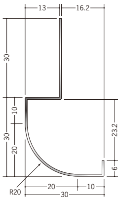
20097 ステン LER-1220 2.73m/ヘアーライン t=0.8mm
