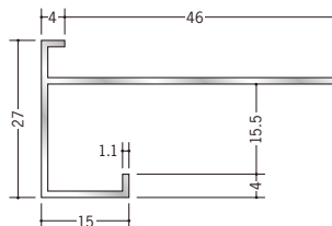
59041 アルミD型44 アクリル焼付 3m / 焼付塗装
