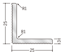
36213 木目アングル25入隅用 2.5m / 枠目調 / 50本入
