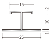
54109 アルミ EH-10 3m/アルマイトシルバー
