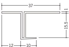
34098 FP-15 1.82m/ホワイト/100本入
