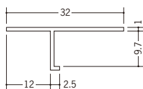
34051 T-9 1.82m/ホワイト/100本入
