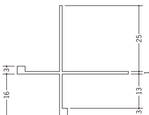
39097 エックスコーナー13+3 2.5m/ホワイト/50本入
