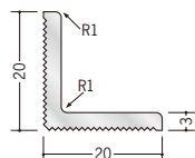
36212 木目アングル20入隅用 2.5m / 枠目調 / 50本入
