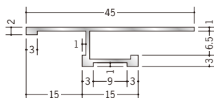
52296 アルミSTB-1506 3m/アルマイトシルバー
