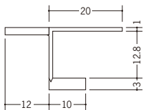
33166 FS-12 テープなし 1.82m/ホワイト/20本入
