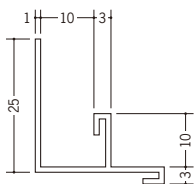
33232 BFX-10 2.73m/ホワイト/50本入
