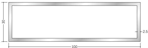
56336 アルミ角パイプ 2.5×30×100 2.5m (-3mm, +5mm) アルマイトシルバー
