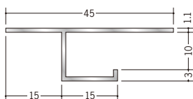
59034 アルミBM-15 アクリル焼付 3m/焼付塗装
