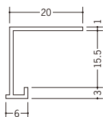
34115 FD-15.5 2m/ホワイト/80本入
