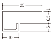
34357 PLG-6 2m/ホワイト/100本入
