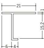
33106 TV-615 1.82m/ホワイト/100本入
