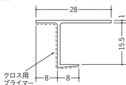
34356 CP-1508 1.82m/ホワイト/100本入
