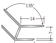
52012 アルミ D135-6 2.73m / アルマイトシルバー
