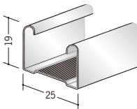
65006 シングルバー19 1.5m・3m / t=0.4~0.45mm 各20本束
