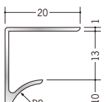
54517 アルミNR-13 2.73m / アルマイトシルバー
