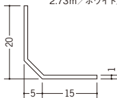
01130 ビニール面取 L20-5M 1.82m/ホワイト/100本入 2.73m/ホワイト/100本入
