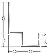
52043 アルミFL-15 3m/アルマイトシルバー
