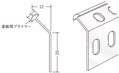
04013 かど定木R-12 プライマー付 1.82m / 半透明 / 150本入
