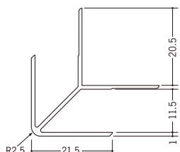
37090 出隅 11 2.5m / ホワイト / 50本入 2.73m / ホワイト / 50本入
