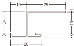
34143 JH-13 2m / ホワイト / 100本入
