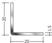
20035 ステンアングル 1.5×20×20 3m/ヘアーライン
