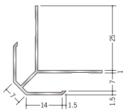
7 53121 アルミ DAM-707 2.73m/アルマイトシルバー
