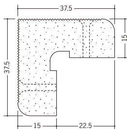
01283 PSコーナー 15mm 2.6m/ミルキー/20本入
