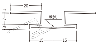
37019 フリージョイナー9 2.5m/ホワイト/50本入
