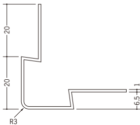
37106 イカ3R-6mm 2.73m/ホワイト/60本入
