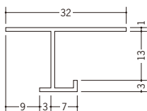
34134 VH-12.5 2m/ホワイト/40本入
