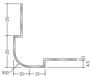
R10 50010 アルミタコ出隅4 2.73m / アルマイトシルバー
