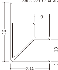
37038 入隅 12 2.5m / ホワイト / 40本入 2.73m / ホワイト / 40本入 3m / ホワイト / 40本入
