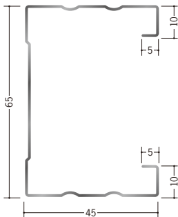
65051 スタット65mm 3m/ t=0.6~0.7mm/ 穴1ヶ所/ 4本束
