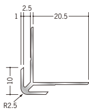
55016 アルミ DA-6.5 2.73m/アルマイトシルバー 3m/アルマイトシルバー
