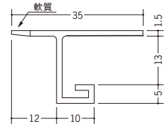
33037 NB-24 2m/ホワイト 100本入
