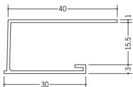
34365 LAW-15 2m/ホワイト/50本入
