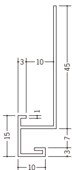
33511 CTX-710 2m/ホワイト/20本入
