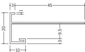
33168 CX-95F (岩綿板用) 2m/ホワイト/40本入
