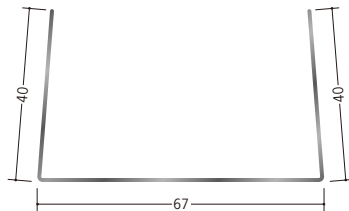
65052 ランナー65mm 1.5m・3m/ t=0.6~0.7mm 各6本束
