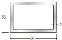
56328 アルミ角パイプ 2×20×30 2.5m (-3mm, +5mm) アルマイトシルバー
