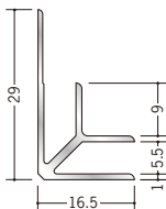
55035 アルミ BF-5.5 2.73m / アルマイトシルバー
