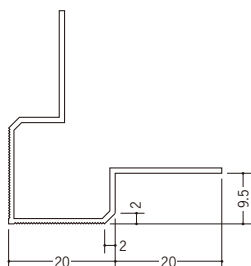
01207 直角コーナー-9.5 2.73m/ホワイト/20本入
