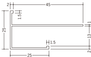
33509 MCX-1225F 2m / ホワイト / 50本入
