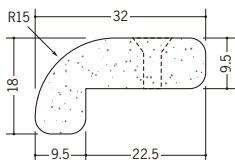
01326 発泡コーナー 15R 9.5 2.6m/ミルキー/50本入
