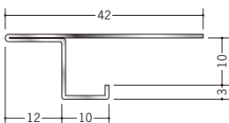
20013 ステン STZ-9 3m/ヘアライン/t=0.8mm
