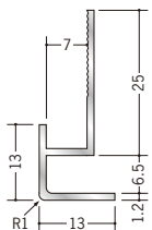
52074 アルミ D型6 2.5m / アルマイトシルバー
