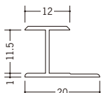
35038 HG-15.5 1.82m/ホワイト/50本入 2.42m/ホワイト/50本入
