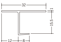
34398 CAP-15 1.82m/ホワイト/100本入
