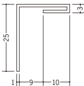
33130 HKS-9 1.82m/ホワイト 100本入
