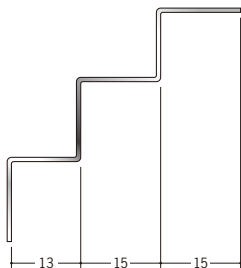
64053 ステン角型入隅 12.5 2.73m/ヘアライン・鏡面 (#800) t=0.8mm
