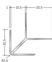
55020 アルミ DA-10.5 2.73m/アルマイトシルバー
