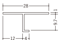
34187 TVC-9 2m/ホワイト/100本入
