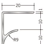
54516 アルミNR-10 2.73m / アルマイトシルバー
