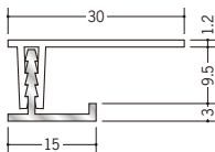
60081 廻り縁KS-15型 アクリル焼付 3m/焼付塗装 ベース (ビニール)/クリーム・グレー・ブラウン
