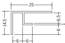
34276 TKF-606 2.73m/ホワイト/50本入
