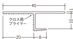
33504 CP-920 1.82m/ホワイト/80本入
