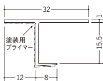
33229 PPZ-15 2m/ホワイト/80本入
