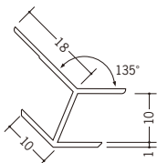
37030 出隅 135°-10 2.5m/ホワイト/50本入 2.73m/ホワイト/50本入
