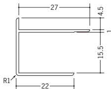
39076 ペンキ出隅 5.5 2.73m/ホワイト/100本入
