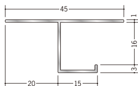
20 51057 アルミ B型16 3m / アルマイトシルバー
