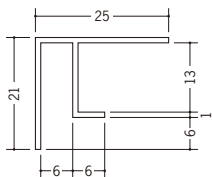
34279 TKF-613 2.73m/ホワイト/50本入
