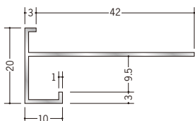
52041 アルミ D 型 31.5 (岩綿板用) 3m / アルマイトシルバー
