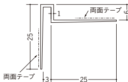
34246 入隅目地3 テープ付 2.5m/ホワイト/80本入 3m/ホワイト/60本入
