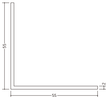
55 36348 アングル 55 (t=2.0) 1.82m/ホワイト/25本入 2.73m/ホワイト/15本入
