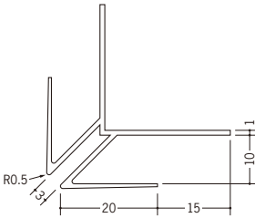
34373 クロス巻き込み出隅10 2.5m/ミルキー/30本入
