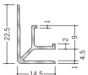
55333 アルミMBF-4.5 2.73m/アルマイトシルバー
