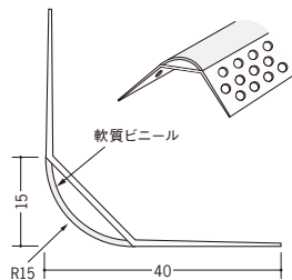
01305 クッションコーナー2型 穴あき 2.5m/ミルキー/50本入
