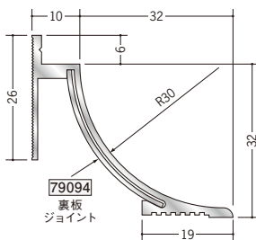
54073 アルミCPB-4 (巾木) 3m/アルマイトシルバー
