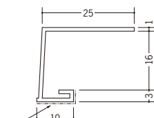
33209 ペンキ見切コ型16 2m/ホワイト/100本入
