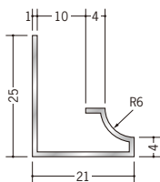
52003 アルミRSA-9 3m / アルマイトシルバー
