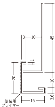
33235 ペンキ見切C-909 2m/ホワイト/50本入
