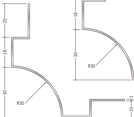
R30 53153 アルミDUM-930 2.73m / アルマイトシルバー
