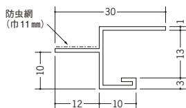
33245 防虫見切 BVB-13A 1.818m / ホワイト / 100本入
