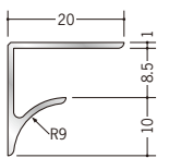
54515 アルミNR-8.5 2.73m / アルマイトシルバー
