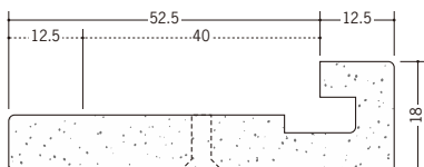
01346 袖壁コーナー 40-12 (12.5mm用) 2.6m/ミルキー/20本入
