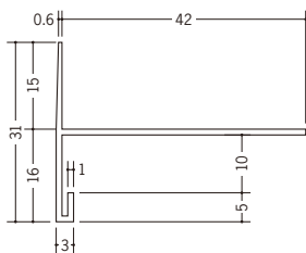
34391 FTX-309 2m/ホワイト/50本入
