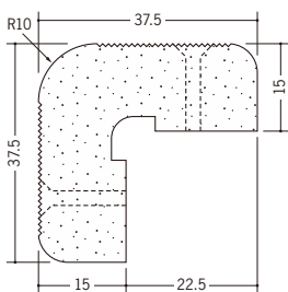
01286 PSコーナー WR 15mm 2.6m/ミルキー/20本入
