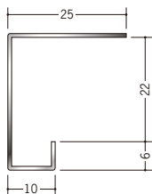
20046 ステン STC-621 3m/ヘア-ライン/t=0.8mm
