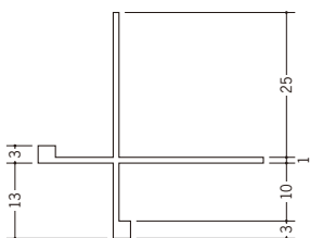
39096 エックスコーナー10+3 2.5m/ホワイト/50本入
