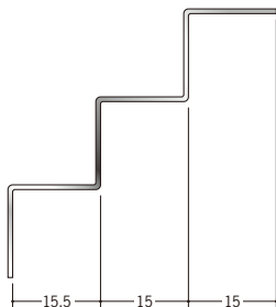
64054 ステン角型入隅 16 2.73m/ヘアライン・鏡面 (#800) t=0.8mm
