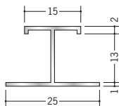
54112 アルミ EH-13 3m/アルマイトシルバー
