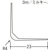
01109 4Rコーナー25 2.5m/ミルキー/100本入 3m/ミルキー/100本入
