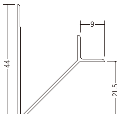
37054 入隅 21 2.5m / ホワイト / 20本入 2.73m / ホワイト / 20本入
