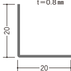
63193 ボンデアングル 0.8×20×20 1.82m / ボンデ鋼板 t=0.8mm
