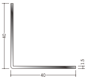
20038 ステンアングル 1.5×40×40 3m/ヘアーライン
