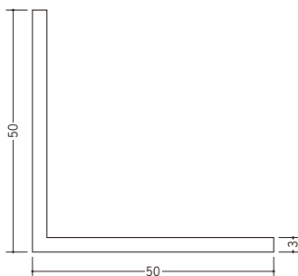
36188 アングル 50 (t=3.0) 1.82m/ホワイト/20本入 2.73m/ホワイト/15本入
