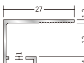
51096 アルミSA-13 3m/アルマイトシルバー
