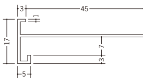
31081 FCX-7M 2m/ホワイト/50本入
