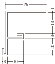
33233 BFX-13 2.73m / ホワイト 50本入
