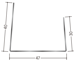
65050 ランナー45mm 1.5m・3m/ t=0.6~0.7mm 各6本束
