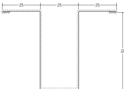
63013 カラー鉄板ハット型51 1.82m/ホワイト・クリーム/t=0.27mm
