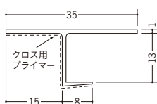
34013 CP-1215 1.82m/ホワイト/100本入
