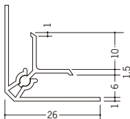
38071 カンゴウジョイナーKI-6.5 2.5m / ホワイト / 30本入
