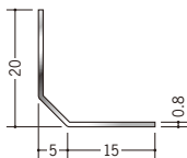
20015 ステン 5mm面取アングル 20 3m/ヘアーライン
