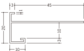
31061 CX-90F 2m/ホワイト/50本入
