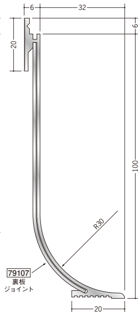
55182 アルミCMR-8 (巾木) 3m/アルマイトシルバー
