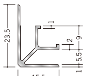
55334 アルミMBF-5.5 2.73m/アルマイトシルバー
