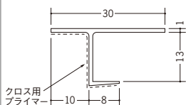
34336 CP-1210 1.82m/ホワイト/100本入
