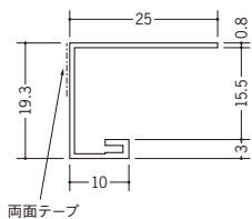
22006 PDW-15 テープ付 2.3m/ホワイト/100本入
