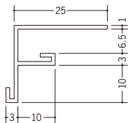
33231 BFX-6.5 2.73m / ホワイト 50本入
