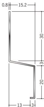
63101 ステン SMK-2 2m/ヘアライン t=0.8mm
