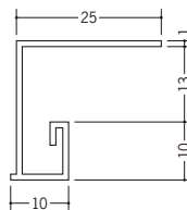
36198 PLM-13 2m/ホワイト/100本入
