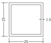
36073 角パイプ25 2m/ホワイト/48本入
