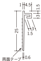
33313 クロス押さえ見切1型-B テープ付 2m/ホワイト/150本入
