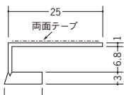
33009 FR-7 テープ付 1.82m/ホワイト/35本入
