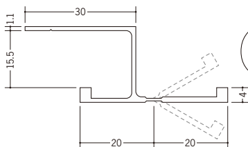
59049 湯らっくす 不燃用フリーボーダー-15 2m / アルミ製 / 焼付塗装
