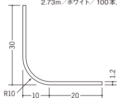
01192 ビニール 10R-30×30 1.82m/ホワイト/100本入 2.73m/ホワイト/100本入
