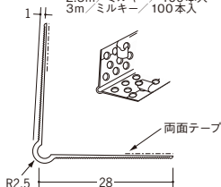
R4 01024 L型コーナー23 2.73m/ミルキー/100本入 3m/ミルキー/100本入
