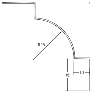
64102 ステン IR-925 2.73m/ヘアライン・鏡面 (#800) t=0.8mm
