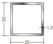
20058 ステン角パイプ 20×20 2.5m/ヘアライン
