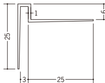
34247 入隅目地3 穴あき 2.5m/ホワイト/80本入 3m/ホワイト/60本入
