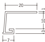
33026 EV-10 1.82m/ホワイト/150本入
