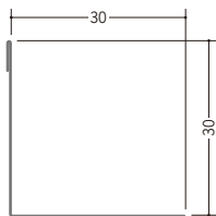
63188 L-30 (外ハゼ) 1.82m / アエンメッキ鋼板 t=0.27mm
