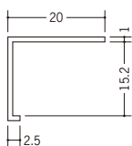
37525 TSC-15 2m/ホワイト/100本入
