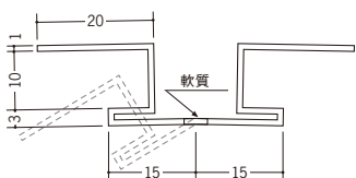
37017 フリージョイナー15 2.5m/ホワイト/30本入
