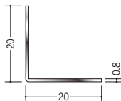
20031 ステンアングル 0.8×20×20 3m/ヘアーライン
