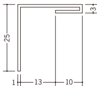
33089 HKS-13 1.82m/ホワイト 100本入
