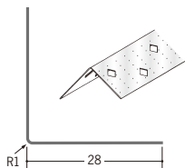
01410 亜鉛折コーナー30×30 2.73m/アエンメッキ鋼板 t=0.35mm
