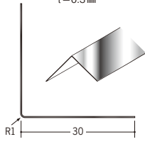
01430 ステン折コーナー30×30 2.73m/±400程度 t=0.3mm
