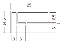
34271 TKF-306 2.73m/ホワイト/50本入
