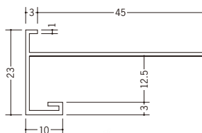
33169 CX-125F (岩綿板用) 2m/ホワイト/40本入
