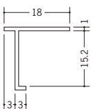
33425 TV-315 1.82m/ホワイト/100本入
