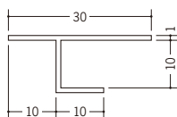
37533 TZT-9 2m/ホワイト/100本入
