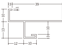
31004 VN-10 2m / ホワイト / 80本入
