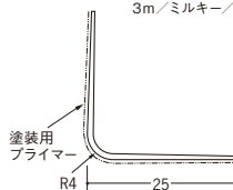
01233 L型コーナー45プライマー付 2.73m/ミルキー/50本入 3m/ミルキー/50本入
