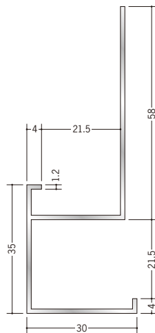
59046 アルミD型26 アクリル焼付 (SK-12・23・30用) 3m / 焼付塗装
