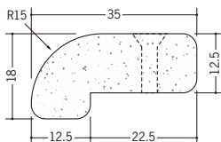
01327 発泡コーナー 15R 12.5 2.6m/ミルキー/40本入
