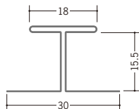
63216 H-15.5 1.82m/アエンメッキ鋼板 t=0.27mm
