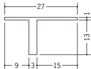
34224 NTX-13 1.82m/ホワイト 50本入
