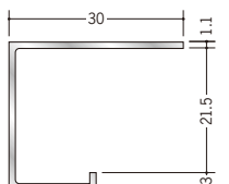
51027 アルミA型20 3m/アルマイトシルバー
