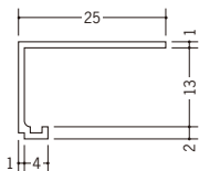
34068 クロスS見切2型 2m/ホワイト/200本入
