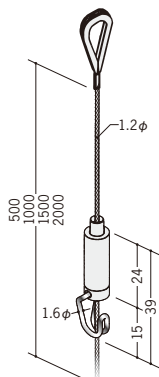
57103 ミニワイヤーハンガー 0.5m/ワイヤー部分ステンレス
