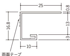
22005 PDW-13 テープ付 2.3m/ホワイト/100本入
