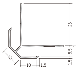
10 53009 アルミ DAM-5 2.73m/アルマイトシルバー
