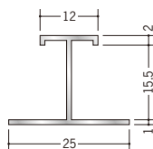
54104 アルミ EHS-15 3m/アルマイトシルバー
