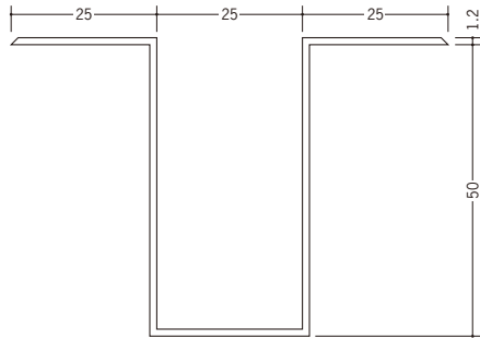
36000 ハット型100 2.73m/ホワイト・クリーム/各10本入
