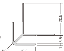
35017 カラー出隅5 2.73m/各50本入 下記全色あり
