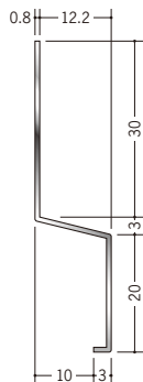
63100 ステン SMK-1 2m/ヘアライン t=0.8mm
