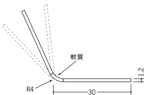
36128 フリーアングル30テープ付 2.5m/ホワイト/60本入
