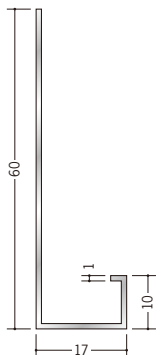
52069 アルミ AFL-13 3m/アルマイトシルバー
