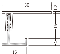
60082 廻り縁KS-20型 アクリル焼付 (SK-12・23・30用) 3m/焼付塗装 ベース (ビニール)/クリーム・グレー・ブラウン
