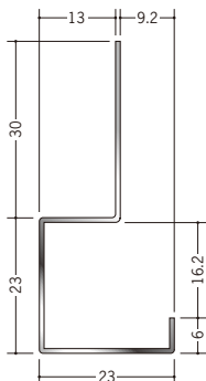
20091 ステン LE-1513 2.73m/ヘアライン t=0.8mm
