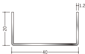
20027 ステンチャンネル 1.2×20×40 3m/ヘアーライン
