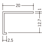
37524 TSC-12 2m/ホワイト/100本入
