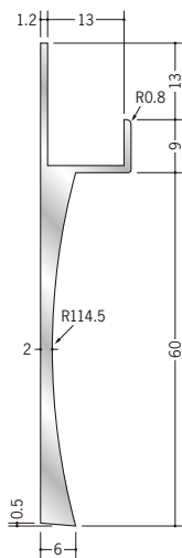
59153 アルミ AFC-1260 2m / アルマイトシルバー
