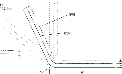
09023 ソフトコーナー50 2.73m/ミルクイー/10本入
