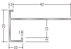
52032 アルミ D 型 32 3m / アルマイトシルバー
