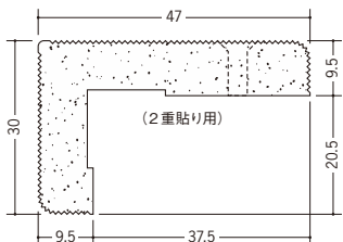
01287 発泡コーナー PBW-9.5 2.6m/ミルキー/20本入
