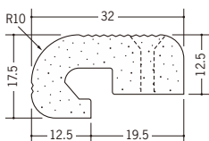
01269 発泡コーナー 10R 12.5mm 2.6m/ミルキー/40本入
