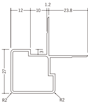
35081 張り出隅10 2.73m/ホワイト/20本入
