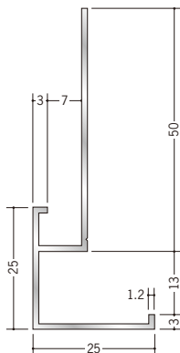
52085 アルミ D型17 3m/アルマイトシルバー
