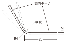
36127 フリーアングル25テープ付 2.5m/ホワイト/75本入
