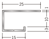
59073 廻り縁15型 アクリル焼付 3m/焼付塗装
