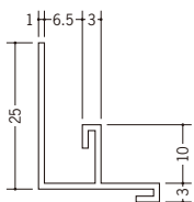
33231 BFX-6.5 2.73m/ホワイト/50本入
