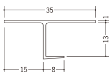
34345 CAP-1215 1.82m/ホワイト/100本入
