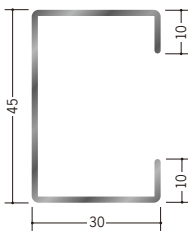
65058 補強材45mm 3m/ t=1.2mm/ 4本束
