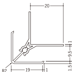
39023 カンゴウジョイナーKD-9 2.5m / ホワイト / 30本入
