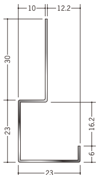
20090 ステン LE-1510 2.73m/ヘアライン t=0.8mm
