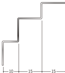
64052 ステン角型入隅 9.5 2.73m/ヘアライン・鏡面 (#800) t=0.8mm
