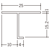
33074 TV-15 1.82m/ホワイト/100本入
