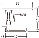
40021 湯らっくす 不燃用開口見切 3m / アルミ製 (ベース: ビニール) 焼付塗装
