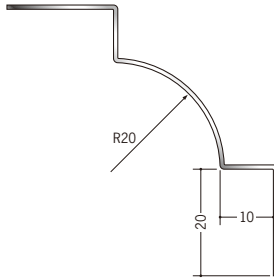
64070 ステン IR-1520 2.73m/ヘアライン・鏡面 (#800) t=0.8mm
