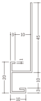
33514 CTX-1010 2m/ホワイト/20本入
