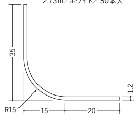
01195 ビニール 15R-35×35 1.82m/ホワイト/100本入 2.73m/ホワイト/50本入
