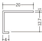
33071 TC-12 1.82m/ホワイト/100本入
