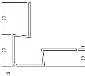
37107 イカ3R-9.5mm 2.73m/ホワイト/60本入
