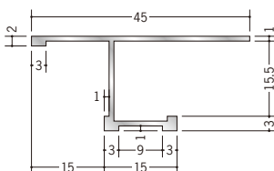
52300 アルミSTB-1515 3m/アルマイトシルバー
