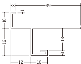
31005 VN-13 2m / ホワイト / 80本入
