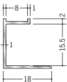
55319 アルミ MCS-15.5 2.73m / アルマイトシルバー
