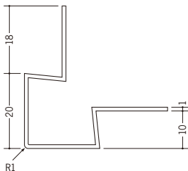
37126 角型イカ出隅10 2.73m/ホワイト/50本入
