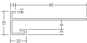
33167 CX-50F 2m/ホワイト/20本入
