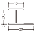
35037 HG-12.5 1.82m/ホワイト/50本入 2.42m/ホワイト/50本入
