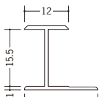
35038 HG-15.5 1.82m/ホワイト/50本入 2.42m/ホワイト/50本入
