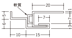
35001 QS-6.5 2m/ホワイト/70本入
