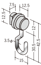
57031 壁フック フック部分ステンレス
