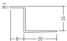
37384 Z-1508 1.82m/ホワイト/100本入
