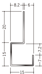
20081 ステン LE-15 2.73m/ヘアライン t=0.8mm
