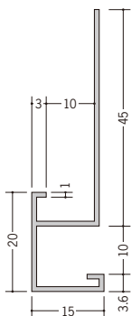
31088 DOL-909 2m/各50本入 下に表記の全色あり
