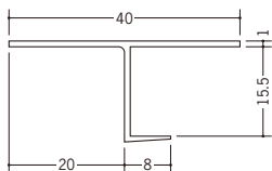
34265 CAP-1520 1.82m/ホワイト/60本入
