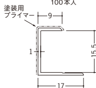
39103 ペンキC型-15.5 2.73m/ホワイト 100本入
