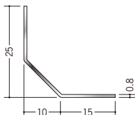
20016 ステン 10mm面取アングル 25 3m/ヘアーライン
