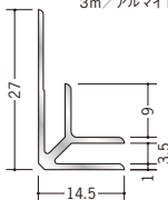
55033 アルミ BF-3.5 2.73m / アルマイトシルバー 3m / アルマイトシルバー
