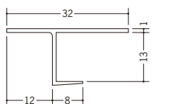
34397 CAP-12 1.82m/ホワイト/100本入
