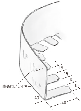
01128 L型コーナーRフリー-40 プライマー付 2.5m/ミルキー/100本入
