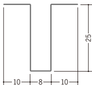
63266 ハット型7号 1.82m/アエンメッキ銅板 t=0.27mm
