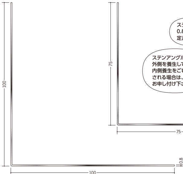
63142 ステンアングル 0.8×100×100 3m/ヘアーライン
