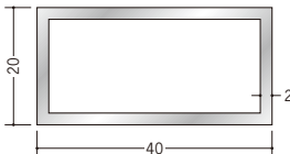
56329 アルミ角パイプ 2×20×40 2.5m (-3mm, +5mm) アルマイトシルバー
