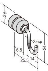
57035 壁用スライドフックB フック部分ステンレス
