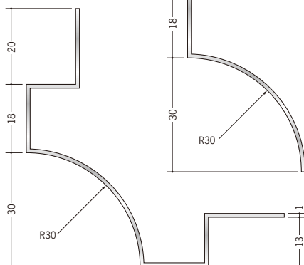
53154 アルミDUM-1230 2.73m / アルマイトシルバー
