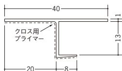
33505 CP-1220 1.82m/ホワイト/70本入
