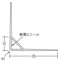
01061 クッションコーナー1型 2.5m/ミルキー/50本入
