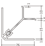
58060 カンゴウAKI-15.5 2.73m / アルマイトシルバー ベース：ビニール
