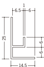
34276 TKF-606 2.73m/ホワイト/50本入
