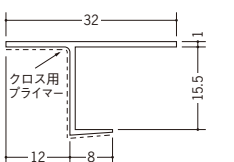
34034 CP-15 1.82m/ホワイト/100本入
