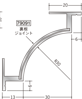
54072 アルミCPB-3 (入隅) 3m/アルマイトシルバー
