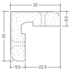
01281 PSコーナー 9.5mm 2.6m/ミルキー/40本入
