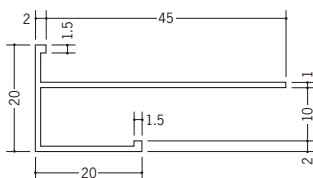
31067 MCX-9F 2m/ホワイト/50本入
