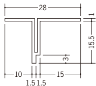
34037 KT-15 1.82m/ホワイト 100本入
