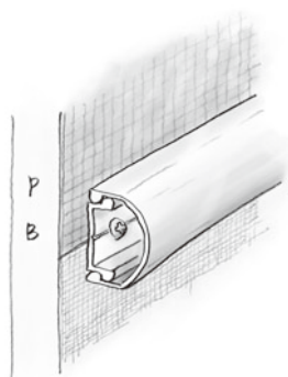
55148 腰かべモール RA-20S用キャップ ビニール / t=1.5mm / シルバーメタリック
