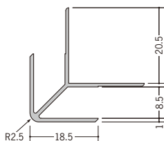
35019 カラー出隅8 2.73m/各50本入 下記全色あり
