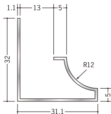
52025 アルミRSB-12.5 3m / アルマイトシルバー
