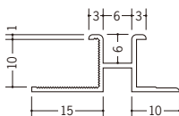
35154 PM-6×10 1.82m/ホワイト 100本入
