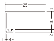
34067 クロスS見切1型 2m/ホワイト/200本入
