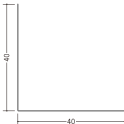
63186 L-40 1.82m / アエンメッキ鋼板 t=0.27mm
