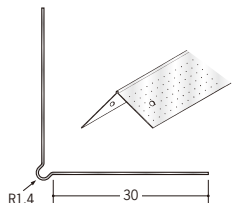
01004 アルミコーナービート30 2.43m/生地材/t=0.4mm
