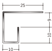
20173 ステン STC-910 3m/ヘア-ライン/t=0.8mm
