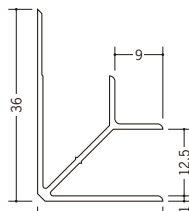
37354 入隅 12B 2.5m / ホワイト / 40本入
