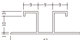
35245 ハット型EAG-10 2.73m / ホワイト / 50本入
