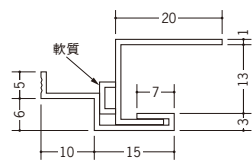
35003 QS-12.5 2m/ホワイト/55本入
