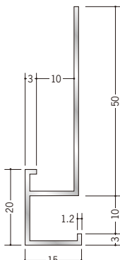
52092 アルミD型22 3m/アルマイトシルバー
