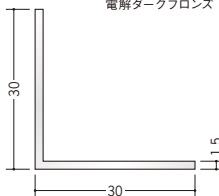
28022 アルミカラーアングル 1.5×30×30BR 3m/電解ステンカラー 電解ライトブロンズ 電解ダークブロンズ
