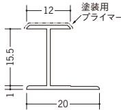
39104 ペンキH型-15.5 2.73m/ホワイト 50本入
