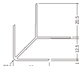
37353 出隅 12B 2.5m / ホワイト / 50本入
