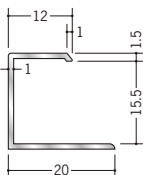
55313 アルミ MCS-4.5 2.73m / アルマイトシルバー
