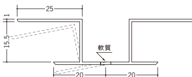
37014 KF-15 2.5m/ホワイト/20本入
