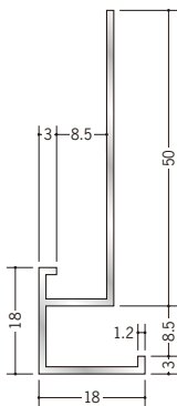
53286 アルミD型47 3m/アルマイトシルバー
