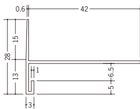
34390 FTX-306 2m/ホワイト/50本入
