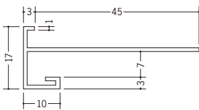
31063 CX-60F 2m/ホワイト/50本入
