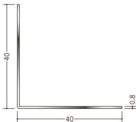
20034 ステンアングル 0.8×40×40 3m/ヘアーライン
