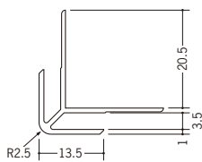
35015 カラー出隅3 2.73m/各100本入 下記全色あり
