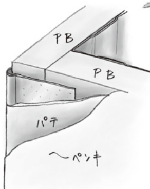
01430 ステン折コーナー30×30 2.73m/±400程度 t=0.3mm
