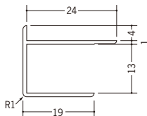
37087 出隅スーパー 12.5 2.5m/ホワイト/50本入 2.73m/ホワイト/50本入
