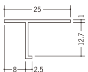
33289 TXV-12 2m/ホワイト/100本入
