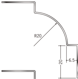
64071 ステン IR-620 2.73m/ヘアライン・鏡面 (#800) t=0.8mm
