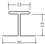
63215 H-13 1.82m/アエンメッキ鋼板 t=0.27mm
