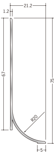
61058 アルミ貼り巾木75-20R 3m/アルマイトシルバー
