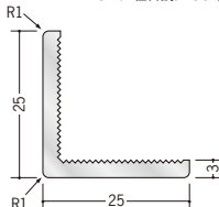
36313 木目アングル25出隅用 2.5m / 枠目調 / 50本入
