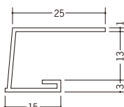
34119 LA-13 2m/ホワイト/100本入
