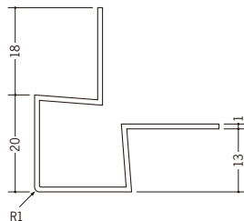
37127 角型イカ出隅13 2.73m/ホワイト/50本入
