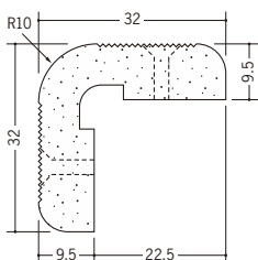
01284 PSコーナー WR 9.5mm 2.6m/ミルキー/40本入
