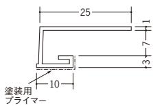
33205 ペンキ見切コ型7 2m/ホワイト/100本入
