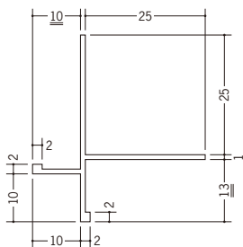
39091 エックスコーナー NT-10 2.5m / ホワイト / 50本入
