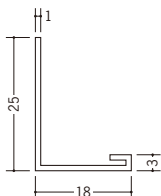
36204 LP-13 2m/ホワイト/100本入
