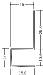
20072 ステン SZ-15 2.73m/ヘアライン t=0.8mm
