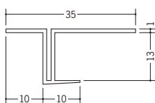
33405 FPZ-13 1.82m/ホワイト/50本入
