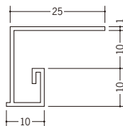
36197 PLM-10 2m/ホワイト/100本入
