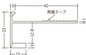
31012 EF-13 テープ付 2m/ホワイト/20本入
