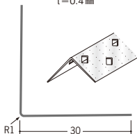
01008 亜鉛角コーナー30 2.73m/アエンメッキ鋼板 t=0.4mm
