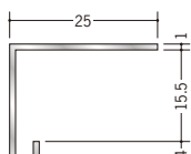
52058 アルミCC15 3m / アルマイトシルバー
