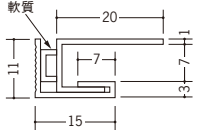
34001 QA-7 2m/ホワイト/80本入
