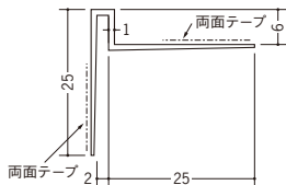
34244 入隅目地2 穴あき+テープ付 2.5m/ホワイト/80本入 3m/ホワイト/60本入
