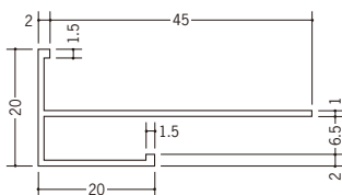
31066 MCX-6F 2m/ホワイト/50本入
