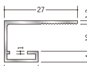
51094 アルミSA-10 3m/アルマイトシルバー
