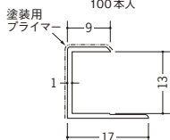
32021 ペンキC型-12.5 2.73m/ホワイト 100本入
