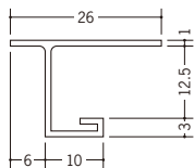
33531 VC-12.5G (岩綿板用) 1.82m / ホワイト 100本入
