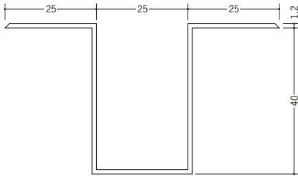
35098 ハット型40 2.73m/ホワイト・クリーム/各25本入
