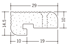
01263 発泡コーナー 9.5mm 2.6m/ミルキー/50本入
