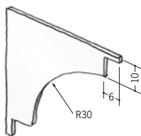
79114 SPB-130 サイドキャップ オフホワイト/1=1.0mm
