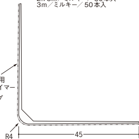
01233 L型コーナー45プライマー付 2.73m/ミルキー/50本入 3m/ミルキー/50本入
