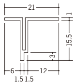
34037 KT-15 1.82m/ホワイト 100本入
