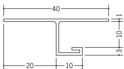
33249 換気見切 KMK-10 1.818m / ホワイト / 50本入 / 開口率11.96%
