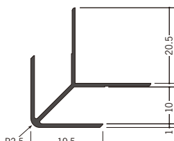
35020 カラー出隅9 2.73m/各50本入 下記全色あり
