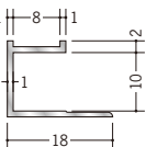
55317 アルミ MCS-10 2.73m / アルマイトシルバー
