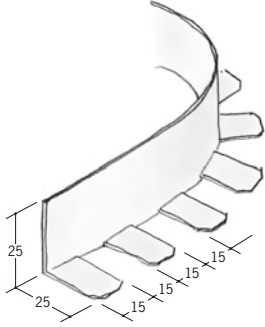
25 01091 L型コーナーRフリー-25 2.5m/ミルキー/100本入
