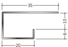
20164 ステン STC-1020 3m/ヘアライン/t=0.8mm
