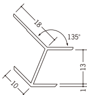
37031 出隅 135°-13 2.5m/ホワイト/50本入 2.73m/ホワイト/50本入
