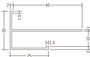
33508 MCX-925F 2m / ホワイト / 50本入
