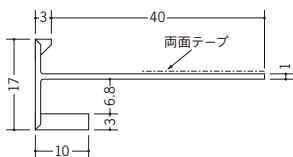
31010 EF-7 テープ付 2m/ホワイト/30本入
