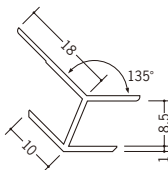
37046 出隅 135°-9 2.5m/ホワイト/50本入 2.73m/ホワイト/50本入
