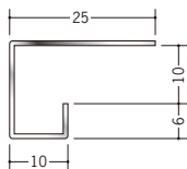
20046 ステン STC-621 3m/ヘア-ライン/t=0.8mm
