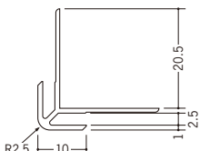
37021 出隅 2 2.5m / ホワイト / 100本入 2.73m / ホワイト / 100本入
