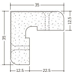
01282 PSコーナー 12.5mm 2.6m/ミルキー/30本入
