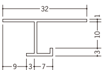
34133 VH-9.5 2m/ホワイト/40本入
