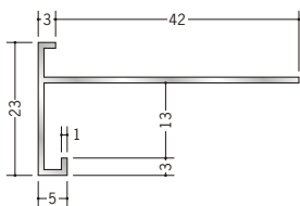
52118 アルミ D型84 3m/アルマイトシルバー
