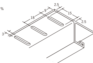
33244 防虫見切 BVB-10A 1.818m / ホワイト / 100本入
