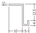
37009 512ZM 2m / ホワイト / 120本入
