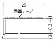
33156 FR-8 テープ付 1.82m/ホワイト/60本入
