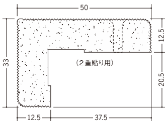
01288 発泡コーナー PBW-12.5 2.6m/ミルキー/12本入
