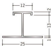
54103 アルミ EHS-12.5 3m/アルマイトシルバー
