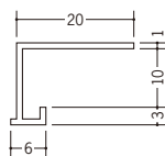
34113 FD-9.5 2m/ホワイト/100本入
