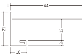
31095 CXK-13F 2m/ホワイト/50本入
