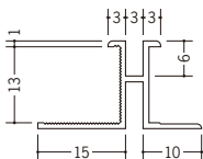
35155 PM-6×13 1.82m/ホワイト 100本入
