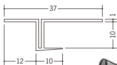
34063 FP-9 1.82m/ホワイト/100本入
