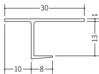
34325 CAP-1210 1.82m/ホワイト/100本入
