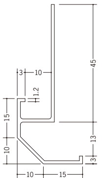
31001 MD-1 2m/ホワイト/40本入
