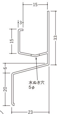
40025 湯らっくす 不燃用水切 3m / アルミ製 焼付塗装
