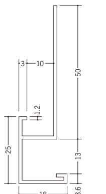
31038 CX-2222 2m/ホワイト/20本入
