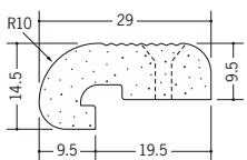
01265 発泡コーナー 10R 9.5mm 2.6m/ミルキー/50本入
