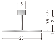
58055 アルミ WBA-512 3m/アルマイトシルバー
