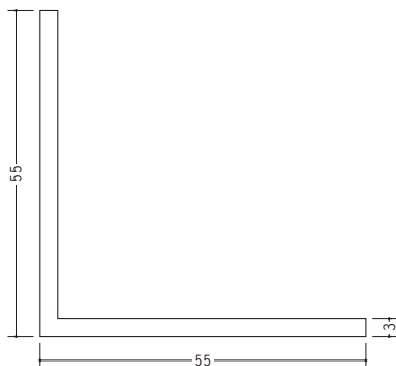
36350 アングル 55 (t=3.0) 1.82m/ホワイト/15本入 2.73m/ホワイト/10本入
