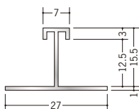
58042 アルミ WBA-715 3m/アルマイトシルバー
