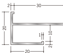
54149 アルミ F 型出隅 9 3m / アルマイトシルバー
