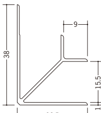
37053 入隅 15 2.5m / ホワイト / 40本入 2.73m / ホワイト / 40本入
