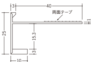
31013 EF-15 テープ付 2m/ホワイト/50本入
