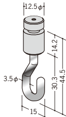
57221 天井用ランナーフック (PR-22F, 33F用) フック部分ステンレス
