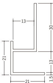
31015 CMX-1313 2m/ホワイト/50本入
