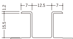
36060 ハット型15 2.5m / ホワイト 50本入
