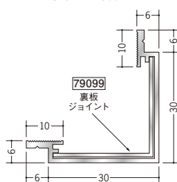
55172 アルミAD-2 (出隅) 3m/アルミトシルバー
