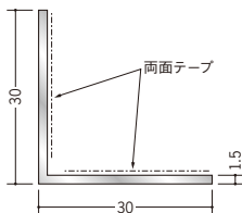
56119 アルミアングル30 テープ付出隅用 3m/アルマイトシルバー
