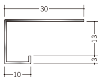
20004 ステン STC-13 3m/ヘア-ライン/t=0.8mm
