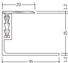
35083 CF-1 (コ型ベース 25mm用) 1.82m / ホワイト / 50本入
