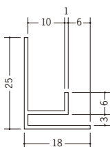
34273 TKF-310 2.73m/ホワイト/50本入
