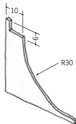
79115 SPB-230 サイドキャップ オフホワイト/1=1.0mm
