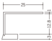
33172 FR-13 テープなし 1.82m/ホワイト/25本入
