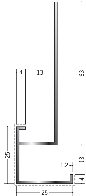
29079 アルミD型17APカラー 3m/バニラホワイト カスタムブラック
