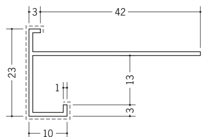
29150 アルミD型32APカラー 3m/バニラホワイト
