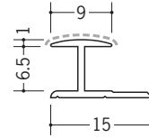
54213 アルミ6HAカラー 2.73m / バニラホワイト カスタムブラック
