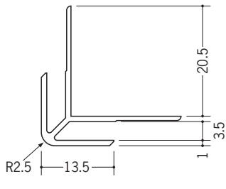
35015 カラー出隅 3 2.73m/各100本入 右ページの全色あり
