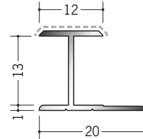
54246 アルミ12.5HS カラー 2.73m / バニラホワイト カスタムブラック
