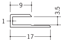
32001 GC-3.5カラー 2.73m/各150本入 右ページの全色あり
