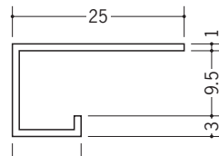
51119 アルミA型12.5BWカラー 3m/ホワイトアルマイト1 電解ブラック
