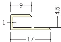
32002 GC-4.5カラー 2.73m/各150本入 右ページの全色あり
