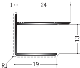
50127 アルミ12ADカラー 2.73m / バニラホワイト カスタムブラック
