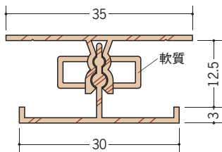
40080 湯らっくす JOH・EOU用ジョイント 2m/ビニール製/オフホワイト・アイボリー ベージュ・ピンク・ブルー・コスモブラック グリーン・ワインレッド・木目調/各40本入
