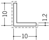
29083 アルミカラーアングル 1.2×10×10 出隅用 3m/パニラホワイト カスタムブラック
