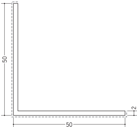
29089 アルミカラーアングル 2×50×50 出隅用 3m/パニラホワイト カスタムブラック
