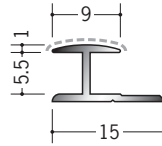
54212 アルミ5HAカラー 2.73m / バニラホワイト カスタムブラック
