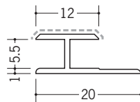
54241 アルミ5.5HS カラー 2.73m / バニラホワイト カスタムブラック
