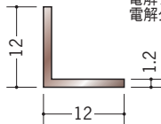
28018 アルミカラーアングル L2R12×12BR 3m/電解ステンカラー 電解ライトブロンズ 電解ダークブロンズ
