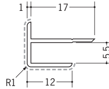
50122 アルミ5ADカラー 2.73m / バニラホワイト カスタムブラック
