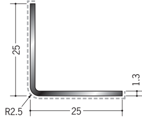
29082 アルミカラーアングル L2R25×25 出隅用 3m/パニラホワイト カスタムブラック
