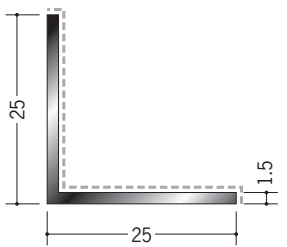
29097 アルミカラーアングル 1.5×25×25入隅用 3m/バニラホワイト カスタムブラック
