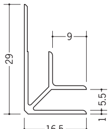
35024 カラー入隅 5 2.73m/各50本入 右ページの全色あり
