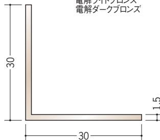
28022 アルミカラーアングル L5R30×30BR 3m/電解ステンカラー 電解ライトブロンズ 電解ダークブロンズ
