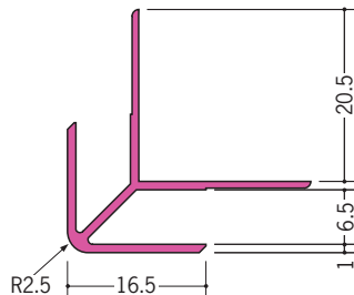
35018 カラー出隅 6 2.73m/各50本入 右ページの全色あり
