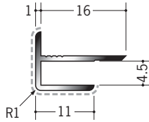
50121 アルミ4ADカラー 2.73m / バニラホワイト カスタムブラック
