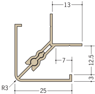
40231 湯らっくす EOU用出隅 3m/ビニール製/オフホワイト・アイボリー ベージュ・ピンク・ブルー・グリーン ワインレッド・木目調/各40本入
