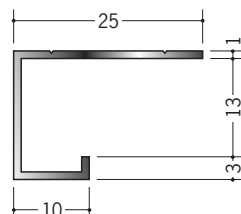
51119 アルミA型12.5BWカラー 3m/ホワイトアルマイト1 電解ブラック
