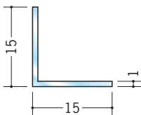
36261 透明アングル15-1 2.5m/透明/100本入
