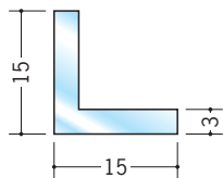
36262 透明アングル15-3 2.5m/透明/50本入
