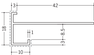
29151 アルミD型33APカラー 3m/バニラホワイト
