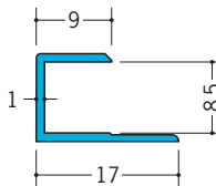
32005 GC-8.5カラー 2.73m/各100本入 右ページの全色あり
