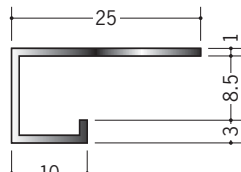
29163 アルミA型12(岩綿板用) BWカラー 3m/ホワイトアルマイト1
