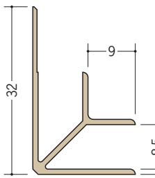
35026 カラー入隅 8 2.73m/各50本入 右ページの全色あり
