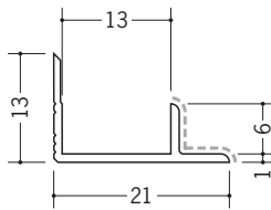
50137 アルミ12ABカラー 2.73m / パニラホワイト カスタムブラック
