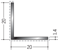
29086 アルミカラーアングル 1.4×20×20 出隅用 3m/パニラホワイト カスタムブラック
