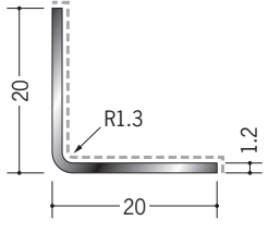
29091 アルミカラーアングル L2R20×20入隅用 3m/バニラホワイト カスタムブラック
