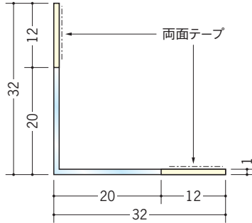
36103 クリアーアングル32テープ付 1.82m/透明+ホワイト・ 透明+アイボリー 各100本入
