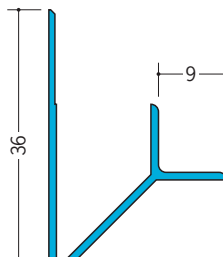
35028 カラー入隅 12 2.73m/各40本入 右ページの全色あり
