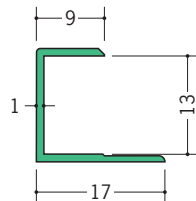
32007 GC-12.5カラー 2.73m/各100本入 右ページの全色あり
