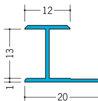
32014 HG-12.5カラー 2.73m/各50本入 右ページの全色あり
