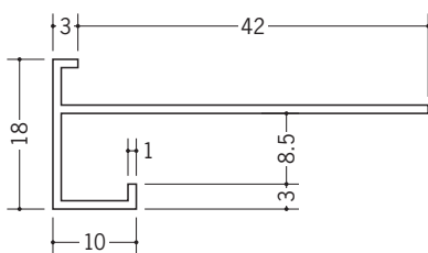
29154 アルミD型33BWカラー 3m/ホワイトアルマイト4
