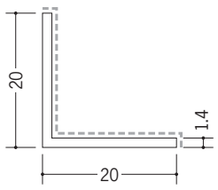
29096 アルミカラーアングル 1.4×20×20入隅用 3m/バニラホワイト カスタムブラック
